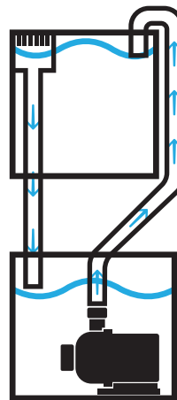
Rückförderpumpe (Als Tauch- oder Inlinepumpe)
