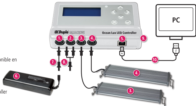
Câble de raccordement
