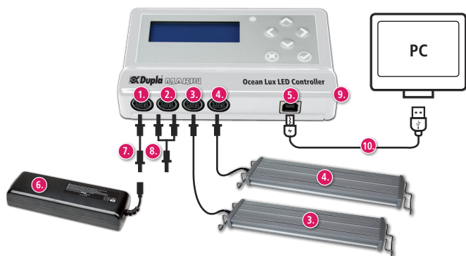
Verbindungskabel
