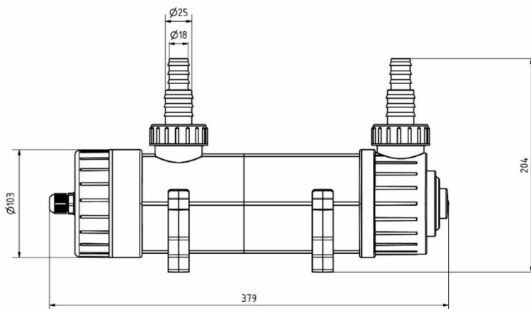
Рис. 3: Размеры Helix Max 18 Вт
