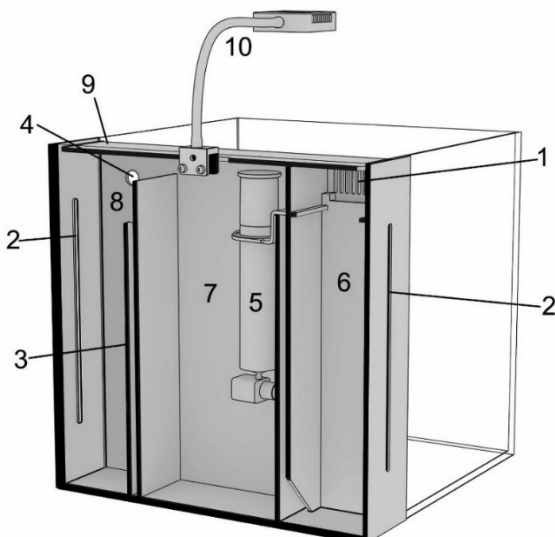
Abb. 1: Filter mit eingehängtem Abschäumer
