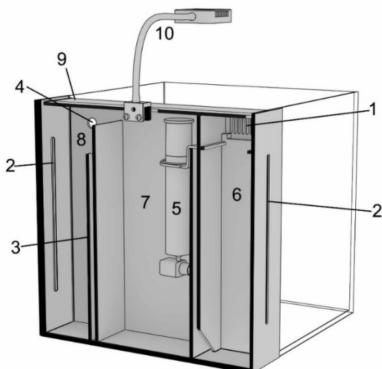
Fig. 1: Filtro con schiumatoio in sospensione
