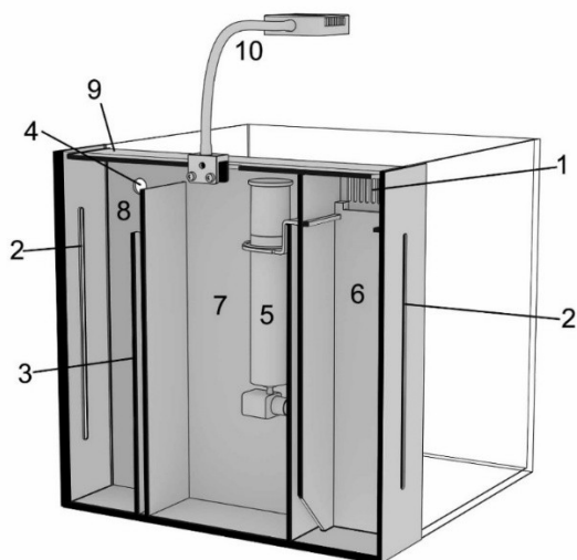
Рис. 2: Фильтр с подвесным скиммером
