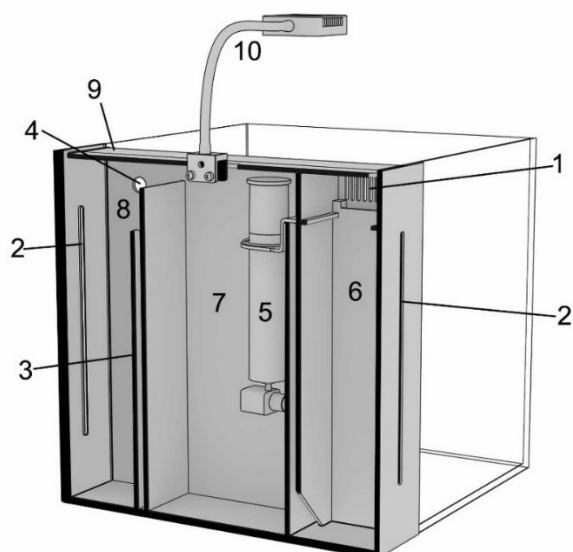
Rys. 1: Filtr z podwieszonym odpieniaczem
