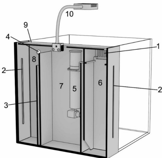
Fig. 1: Filter met hangende afschuimer
