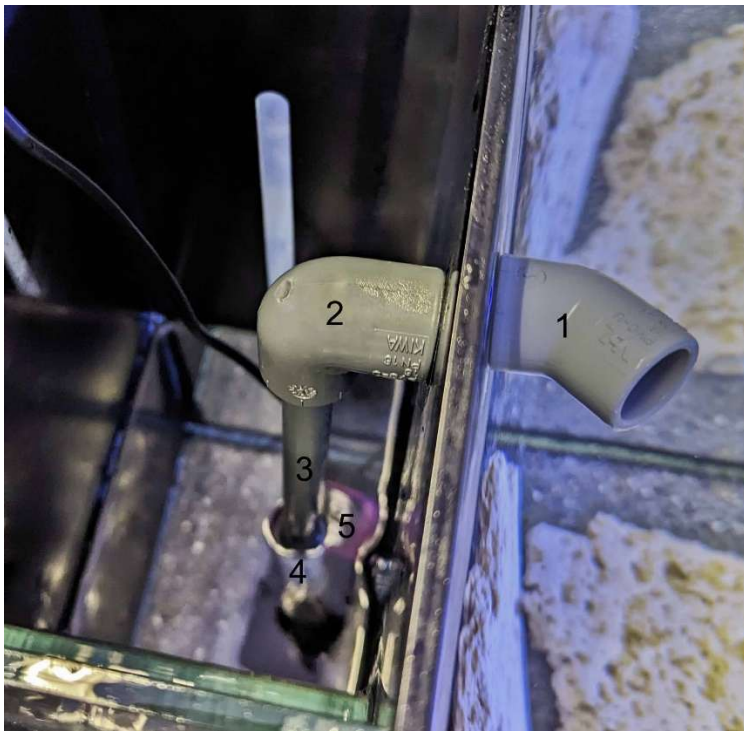
Fig. 3: Montage du DC Runner 600
