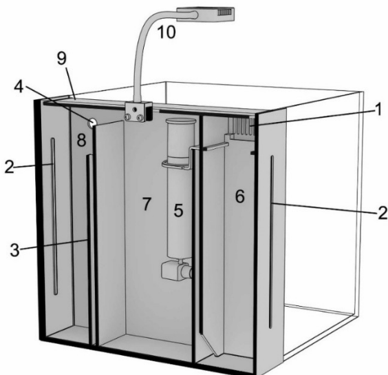
Fig. 1: Filtre avec écumeur suspendu
