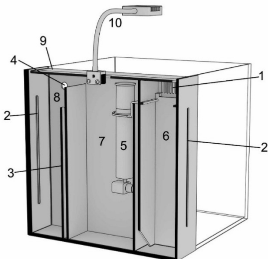
Fig. 1: Filtro con skimmer suspendido
